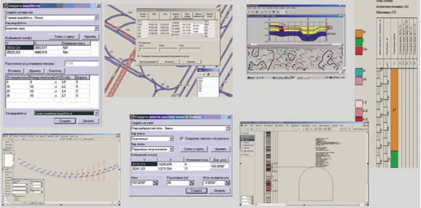
Рис. 2. Примеры реализации задач в подсистеме геолого-маркшейдерского сопровождения горных работ
